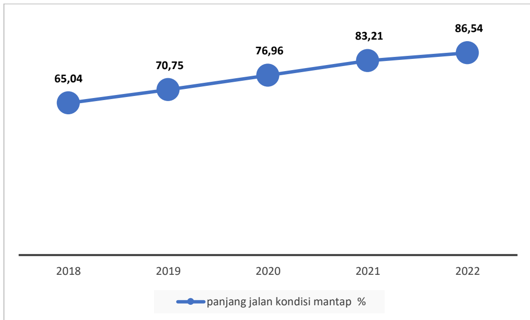
Grafik 2.50 Persentase Panjang Jalan Kabupaten Dalam Kondisi Mantap di Kabupaten Sumedang Tahun 2018-2022
