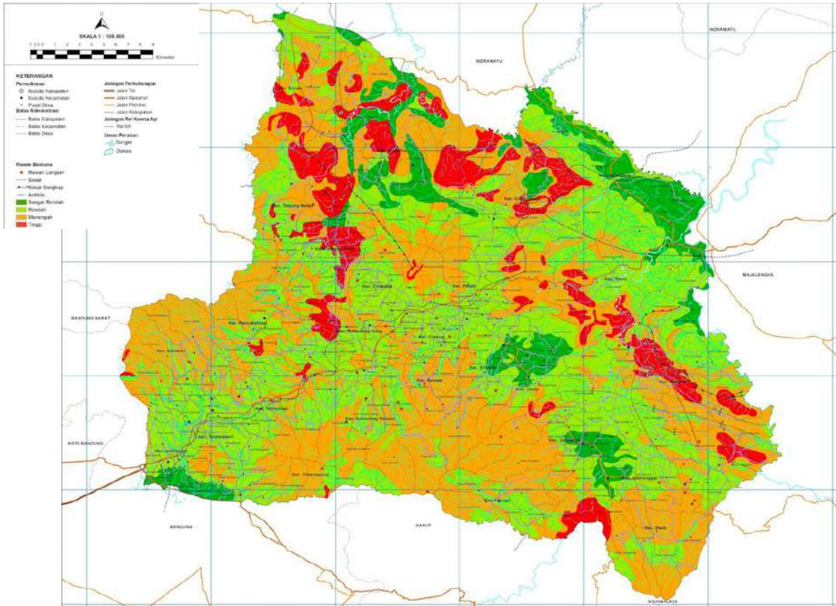
Gambar 2.4 Peta Rawan Bencana Kabupaten Sumedang
